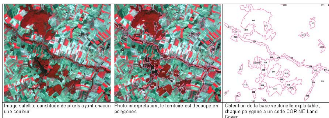
Figure 1-1. Schéma de principe de la photo-interprétation
